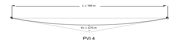
Gambar 4.13. Lengkung Vertikal 4 (PVI 4)
