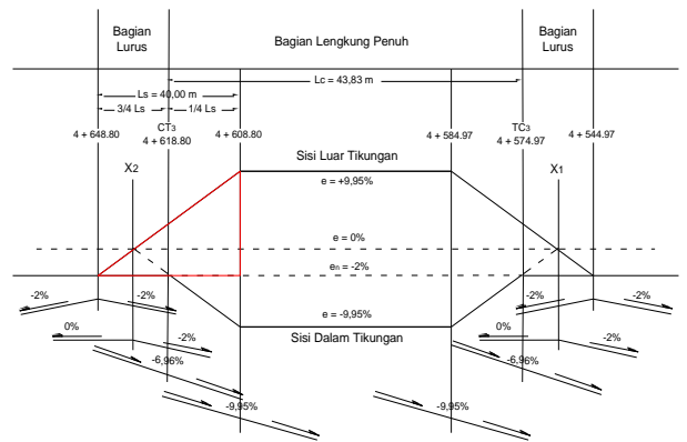
Gambar 4.8. Diagram Superelevasi FC Lengkung P3
