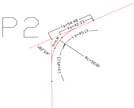
Gambar 4.4. Jenis Tikungan S-C-S Pada Titik P2
