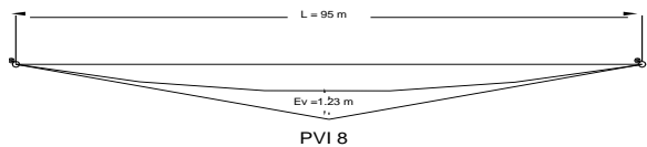
Gambar 4.17. Lengkung Vertikal 8 (PVI 8)
