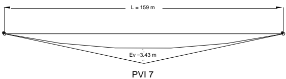
Gambar 4.16. Lengkung Vertikal 7 (PVI 7)
