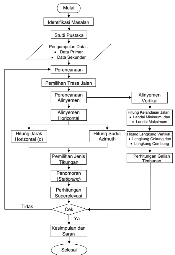
Gambar 1.1. Kerangka Pemikiran
