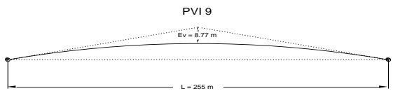
Gambar 4.18. Lengkung Vertikal 9 (PVI 9)
