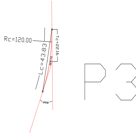
Gambar 4.5. Jenis Tikungan FC Pada Titik P3
