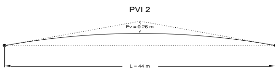
Gambar 4.11. Lengkung Vertikal 2 (PVI 2)
