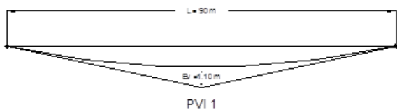
Gambar 4.10. Lengkung Vertikal 1 (PVI 1)
