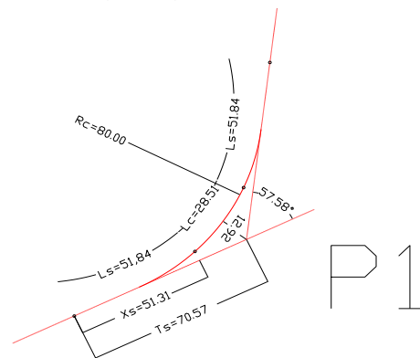
Gambar 4.3. Jenis Tikungan SCS Pada Titik P1
