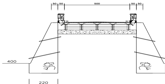
Gambar 4.19. Tipikal Jembatan
