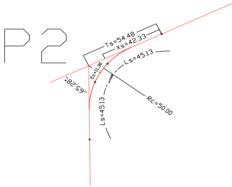
Gambar 4.3. Jenis Tikungan SCS Pada Titik P1
