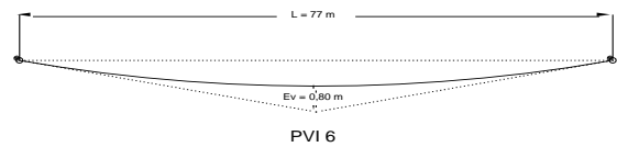
Gambar 4.15. Lengkung Vertikal 6 (PVI 6)
