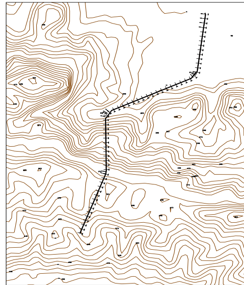
Gambar 4.1. Trase Jalan Rencana
