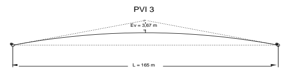
Gambar 4.12. Lengkung Vertikal 3 (PVI 3)
